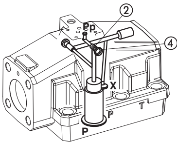
SDPZE-6 控制油路结构
