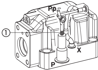
SDPZE-4 控制油路结构
