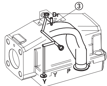
泄油路结构
