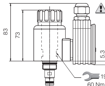
CART SRZME-A (配数字式放大器E-MI-AS-IR)
