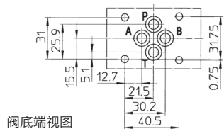
阀底端视图
