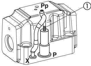
SDPZE-2 控制油路结构
